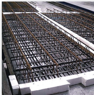
Elementos estructurales preparados para el vertido de hormigón
